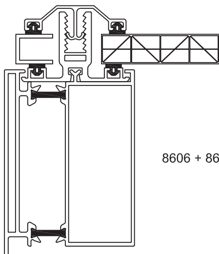
Randprofiel / poteur latéral
