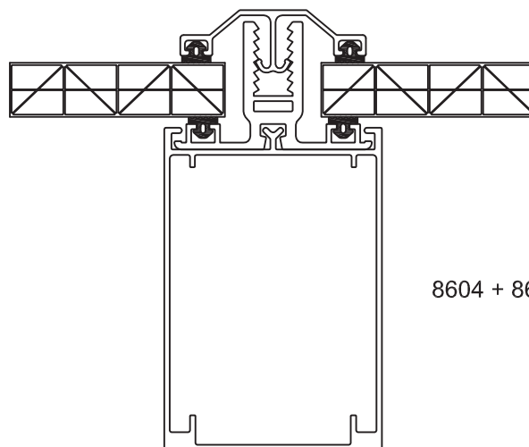
Draagprofiel / Porteur
