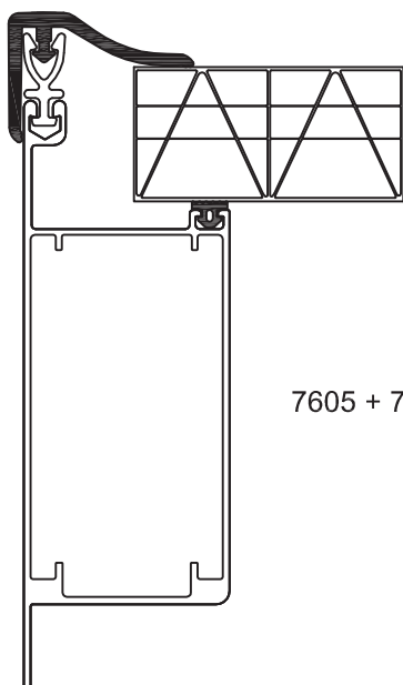
Randprofiel / Porteur latéral
