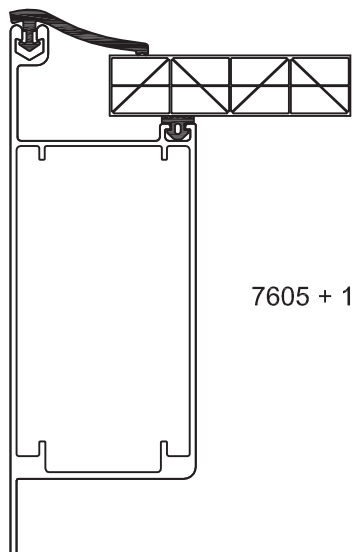
Randprofiel / Porteur latéral
